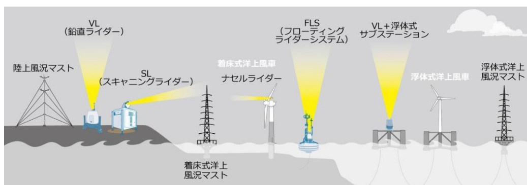
図4 風況観測機器の概略図(本試験サイトにない機器も図の中に含まれます)
